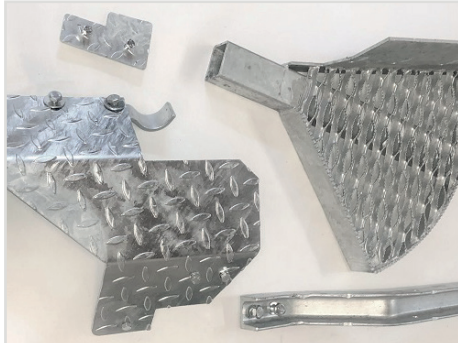
Lieferumfang: Bei Auspuff nach unten: Tritthalter, Trittplatte, Schutzblech, Auspuffschelle, Schraubensatz
